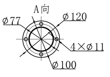
⑤ 消声器排气法兰 Muffler flange
