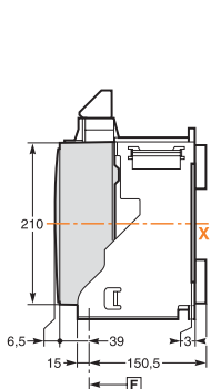
Выключатели Masterpact NT06-NT16, 3/4 – полюсный стационарный аппарат
