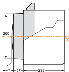
Выключатели Masterpact NW08-NW32, 3/4 – полюсный стационарный аппарат
