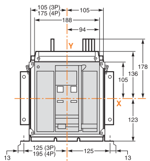
Выключатели Masterpact NT06-NT16, 3/4 – полюсный стационарный аппарат
