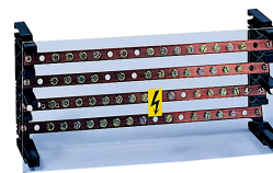
Ступенчатые распределительные блоки
