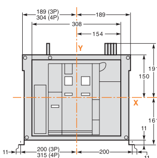
Выключатели Masterpact NW08-NW32, 3/4 – полюсный стационарный аппарат
