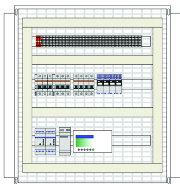
Рис 2.2 Внешний вид блока управления типа «ABP.SE2*-БУ01(03)»
