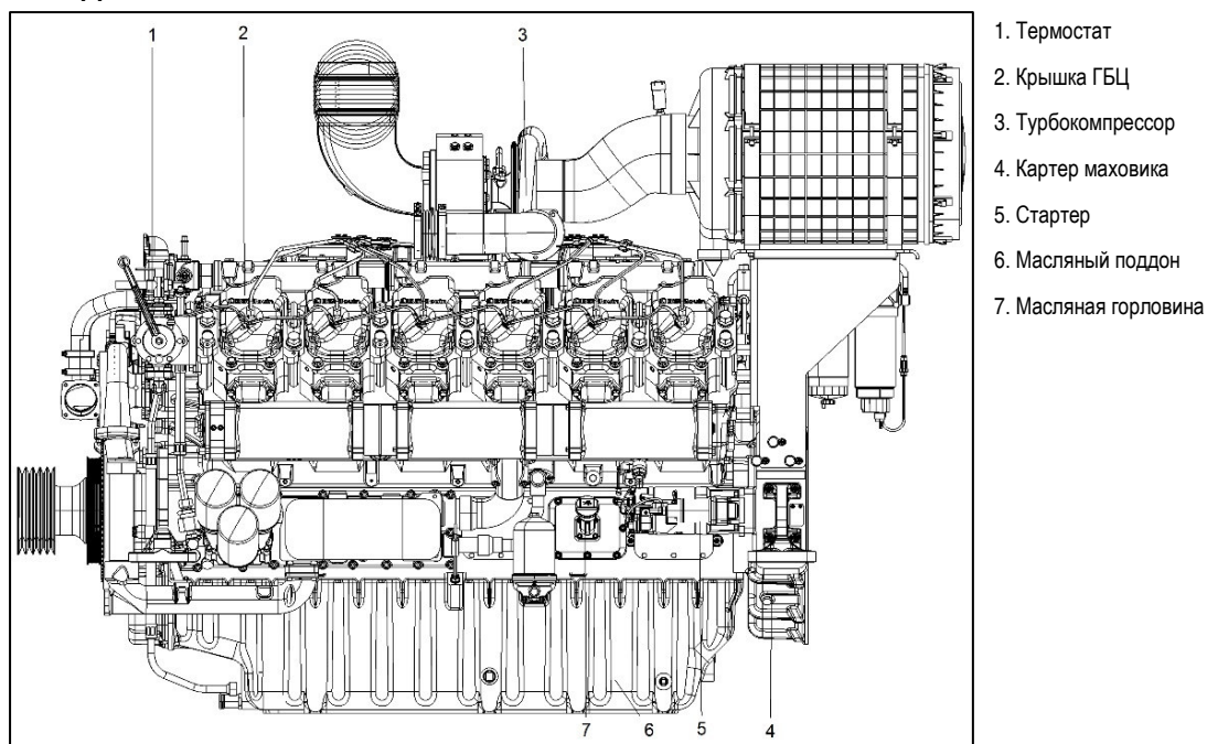
Рисунок 2.3.3А – Вид слева
