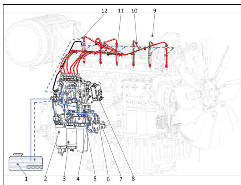
Рисунок 2.6.2 - Схематичное представление топливного контура двигателя 6М33МР
