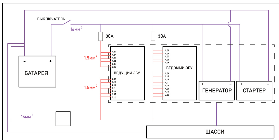
Рисунок 2.7.2Е – Подключение ЭБУ к аккумуляторной батарее
