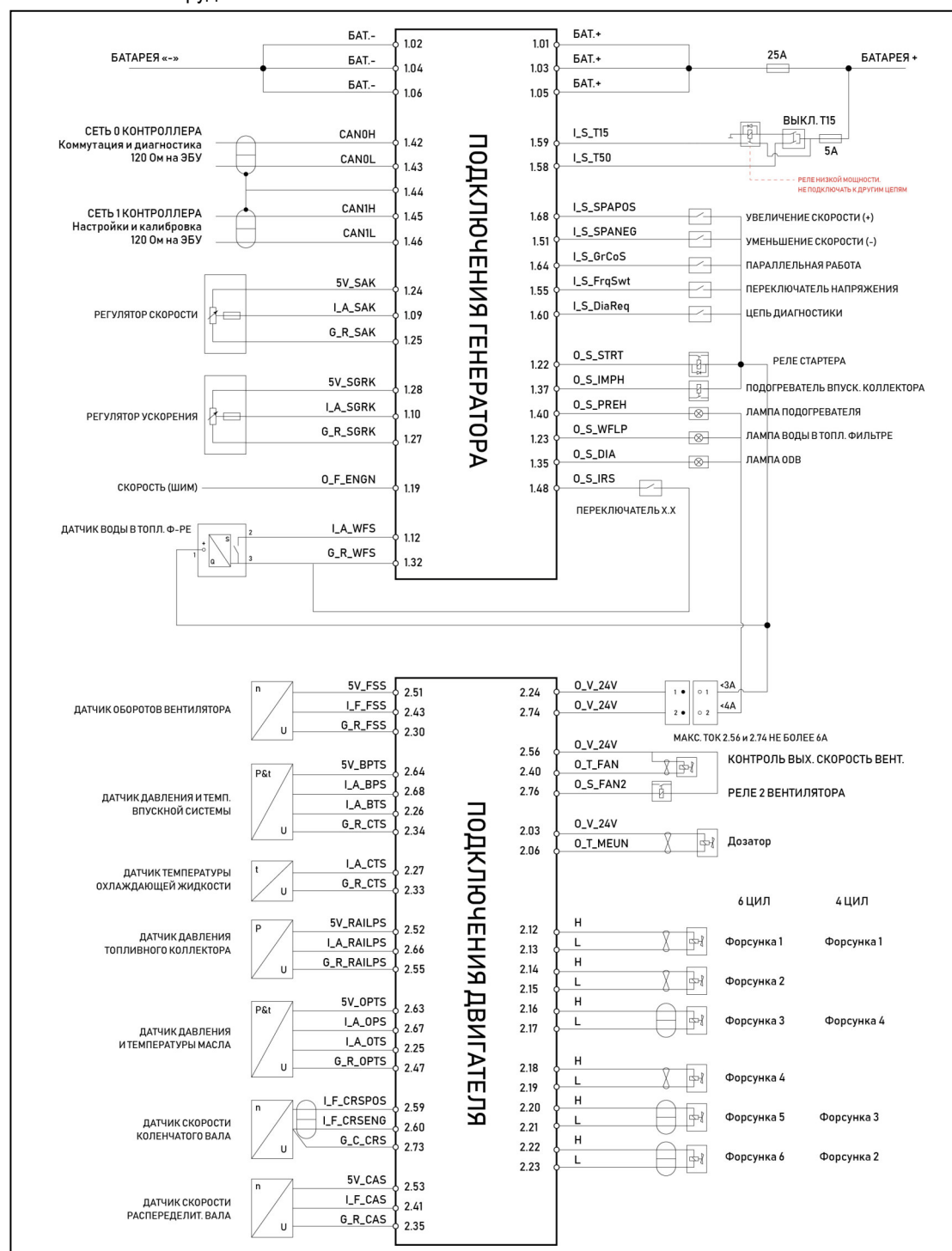
Рисунок 2.7.1А – Электрическая схема подключения ЭБУ WISE15-P160 двигателя 6М33СR
