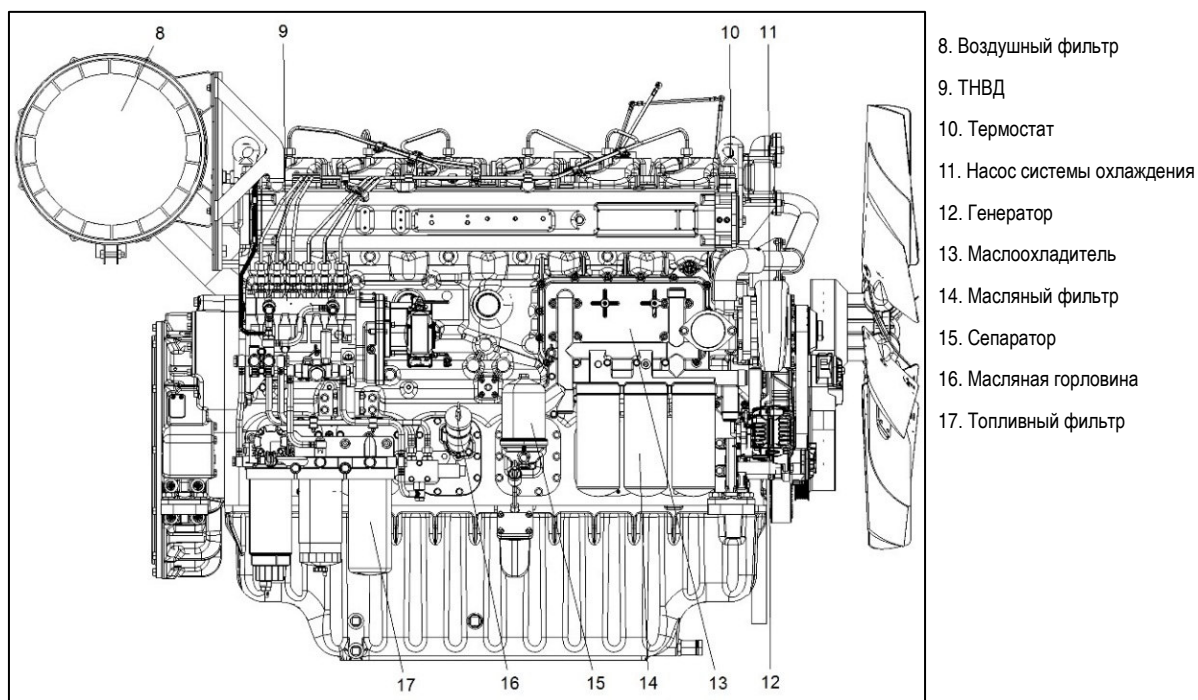
Рисунок 2.3.2В – Вид справа
