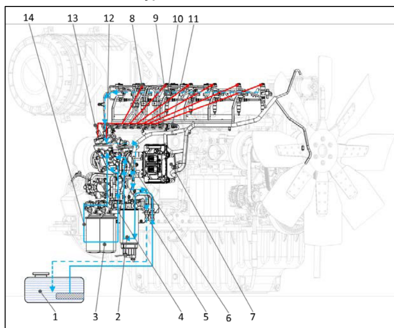
Рисунок 2.6.1 - Схематичное представление топливного контура двигателя 6М33СR
