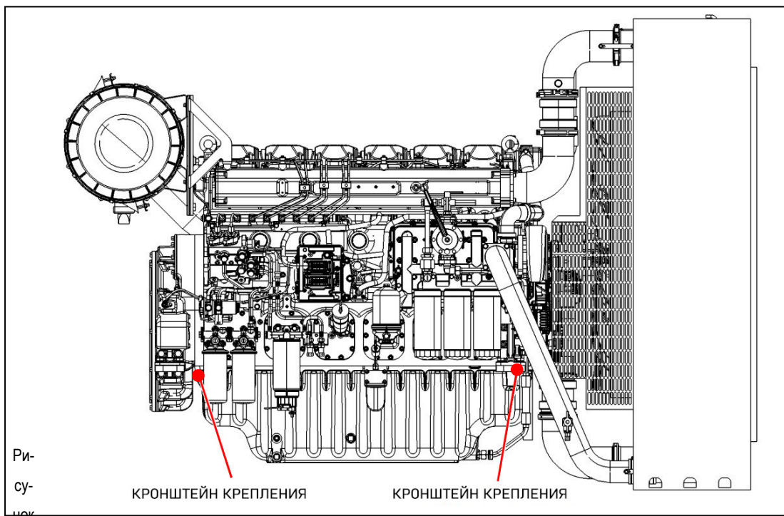
3.2А – Точки крепления 6М33СР
