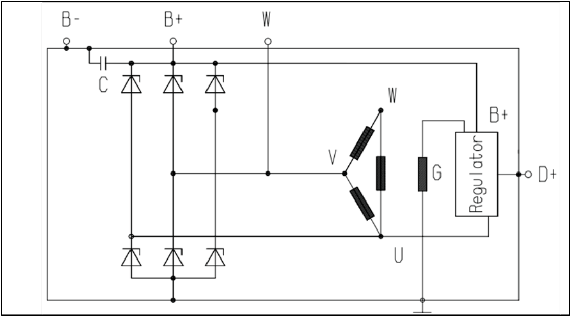
Рисунок 3.9.2В -Электрическая цепь подзаряда аккумулятора двигателя 16М33CR
