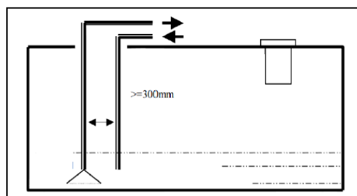
Рисунок 3.8.2 – Топливные контуры
