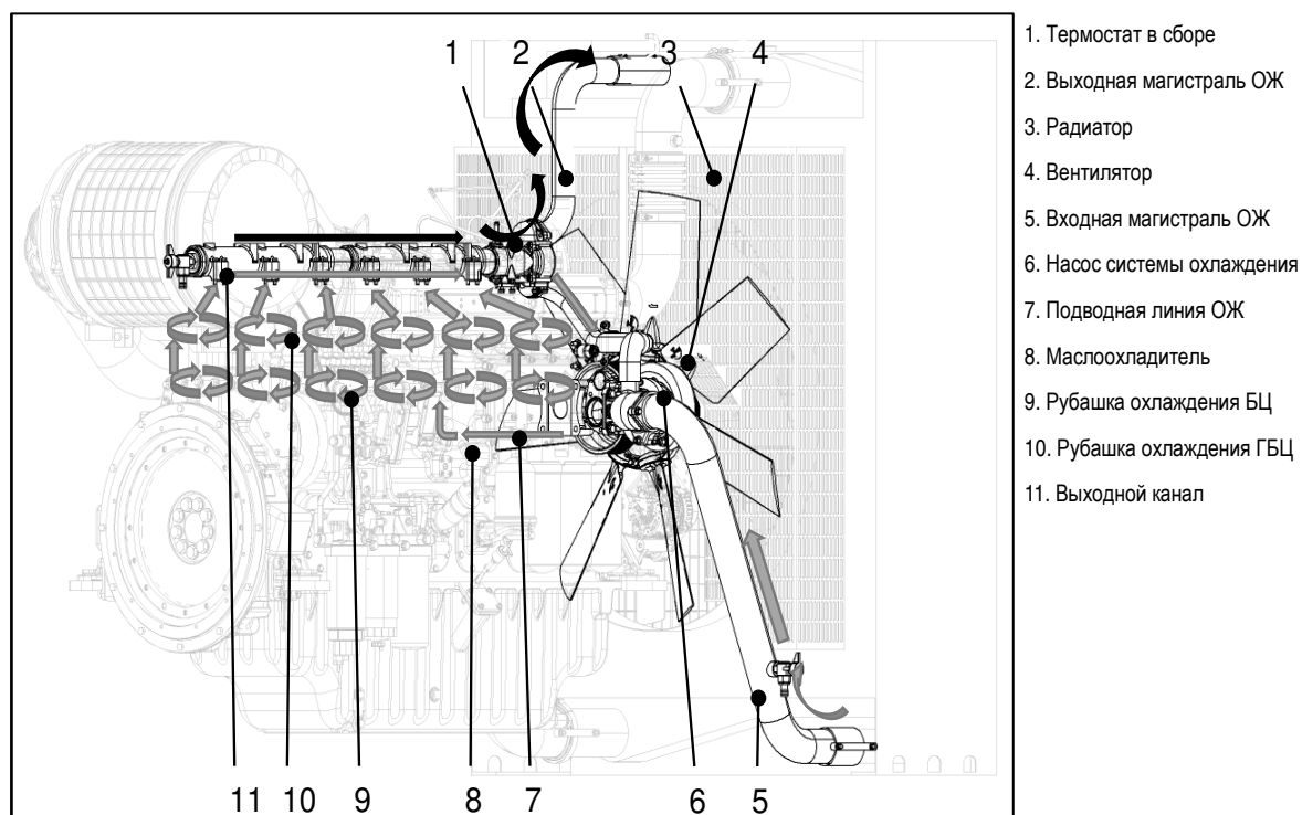
Рисунок 2.4.1 – Схематическое представление контуров охлаждения двигателя 6М33
