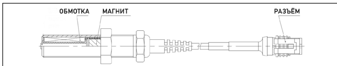
Рисунок 2.8.4А – Конструкция датчика скорости
