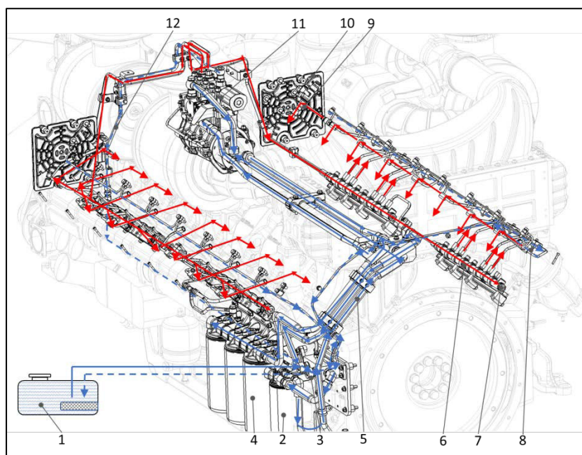
Рисунок 2.6.4 - Схематичное представление топливного контура двигателя 16M33CR
