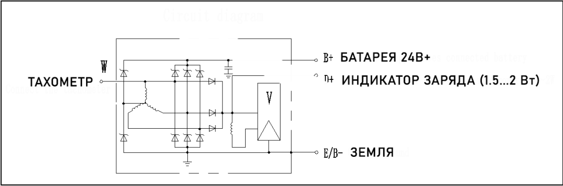
Рисунок 3.9.2А – Электрическая цепь подзаряда аккумулятора двигателя 6М33CR
