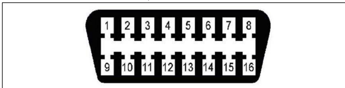
Рисунок 2.7.1М – Внешний вид разъёма
