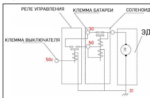
Рисунок 3.9.1А – Подключение стартера 6МЗ3СР
