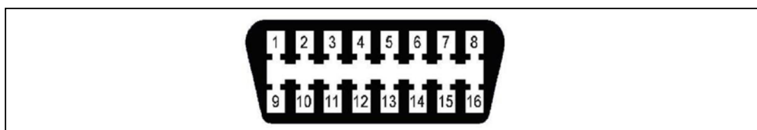
Рисунок 2.7.1I – Внешний вид разъёма
