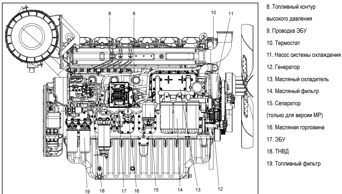
Рисунок 2.3.1В – Вид справа
