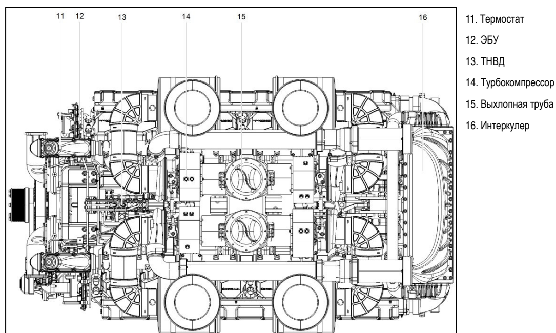
Рисунок 2.3.4В – Вид сверху
