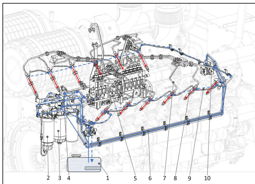
Рисунок 2.6.3 - Схематичное представление топливного контура двигателя 12M33MP
