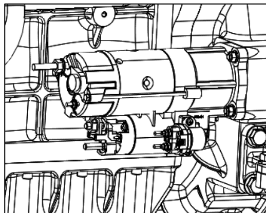
Рисунок 2.7.2G – Стартер
