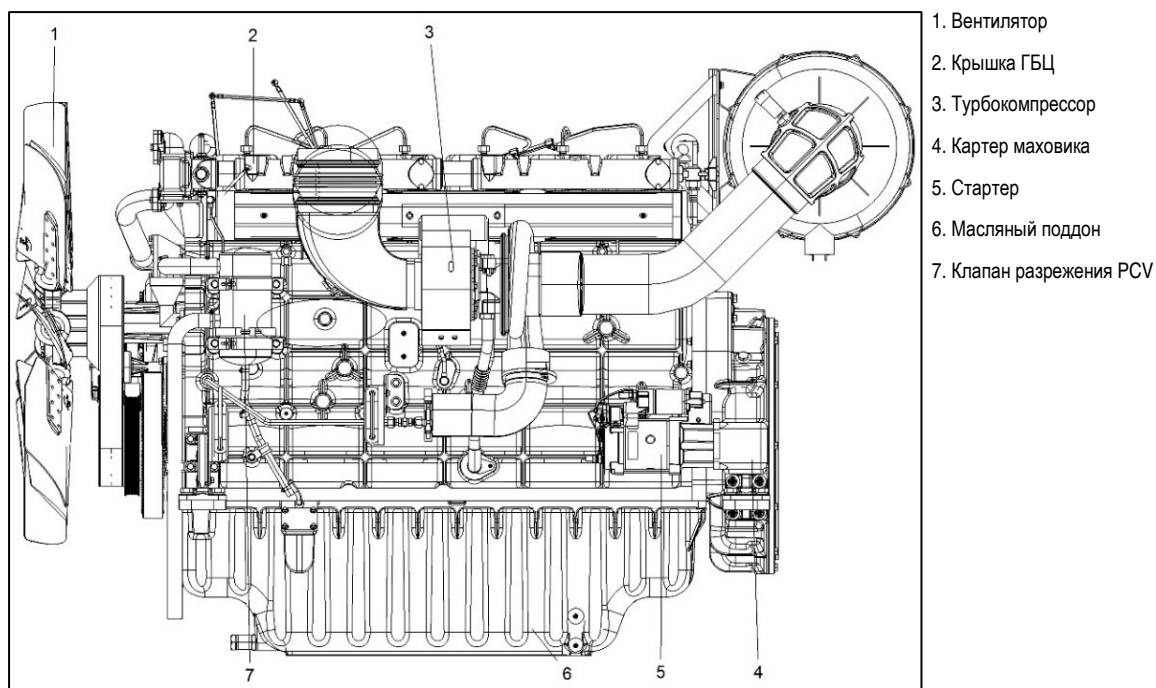
Рисунок 2.3.2А – Вид слева
