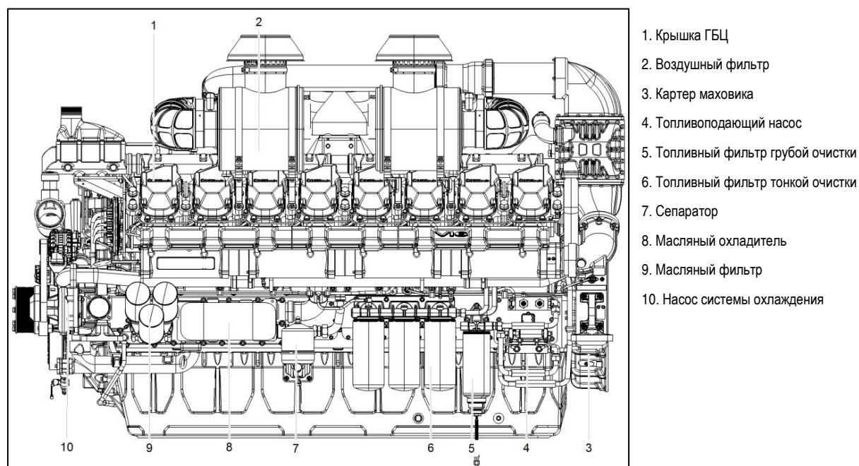
Рисунок 2.3.4А – Вид слева
