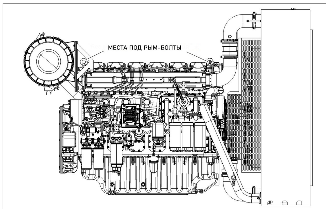
Рисунок 3.1.3А – Двигатель 6МЗЗСР
