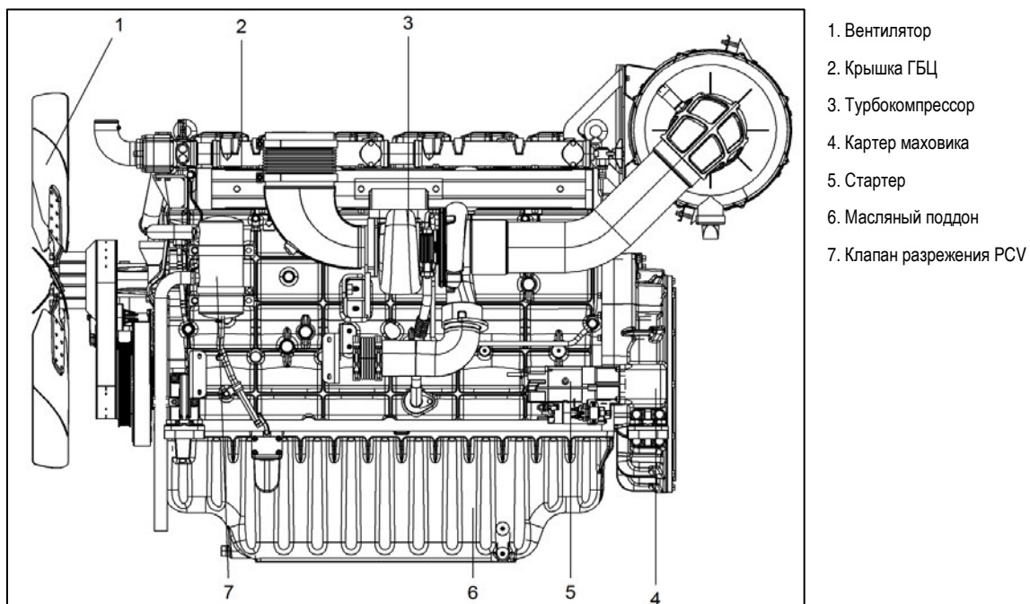
Рисунок 2.3.1А – Вид слева
