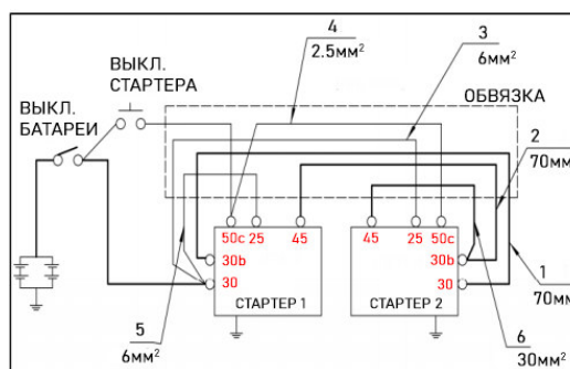
Рисунок 3.9.1В - Подключение стартера 16M33CR
