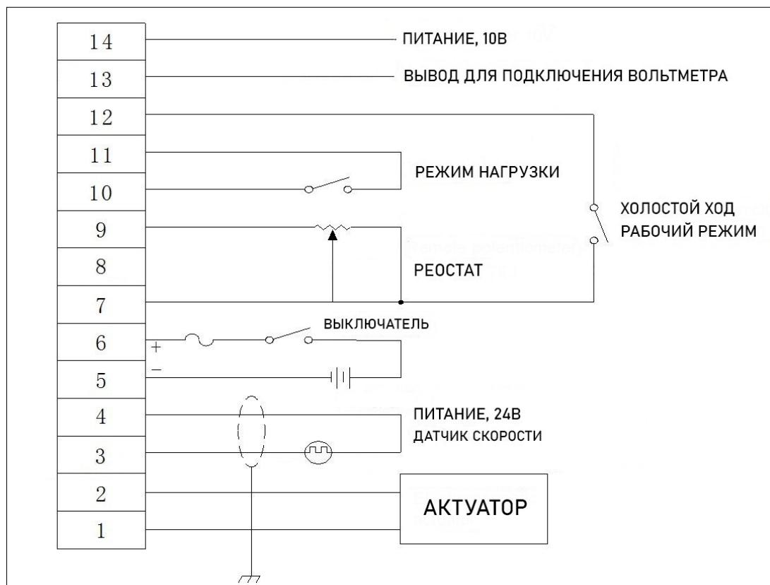
Рисунок 3.11.1В – Схема подключения контроллера C2002
