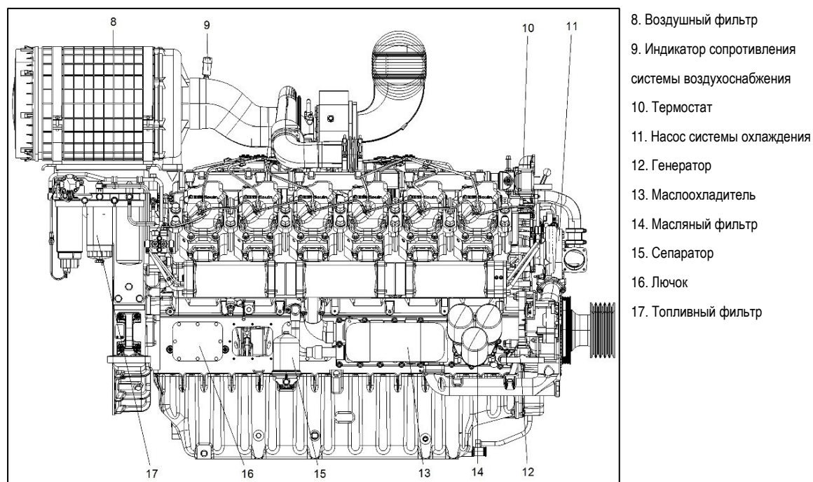
Рисунок 2.3.3В – Вид справа
