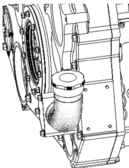
Рисунок 6-4: отверстие для заливки масла и масляный щуп
