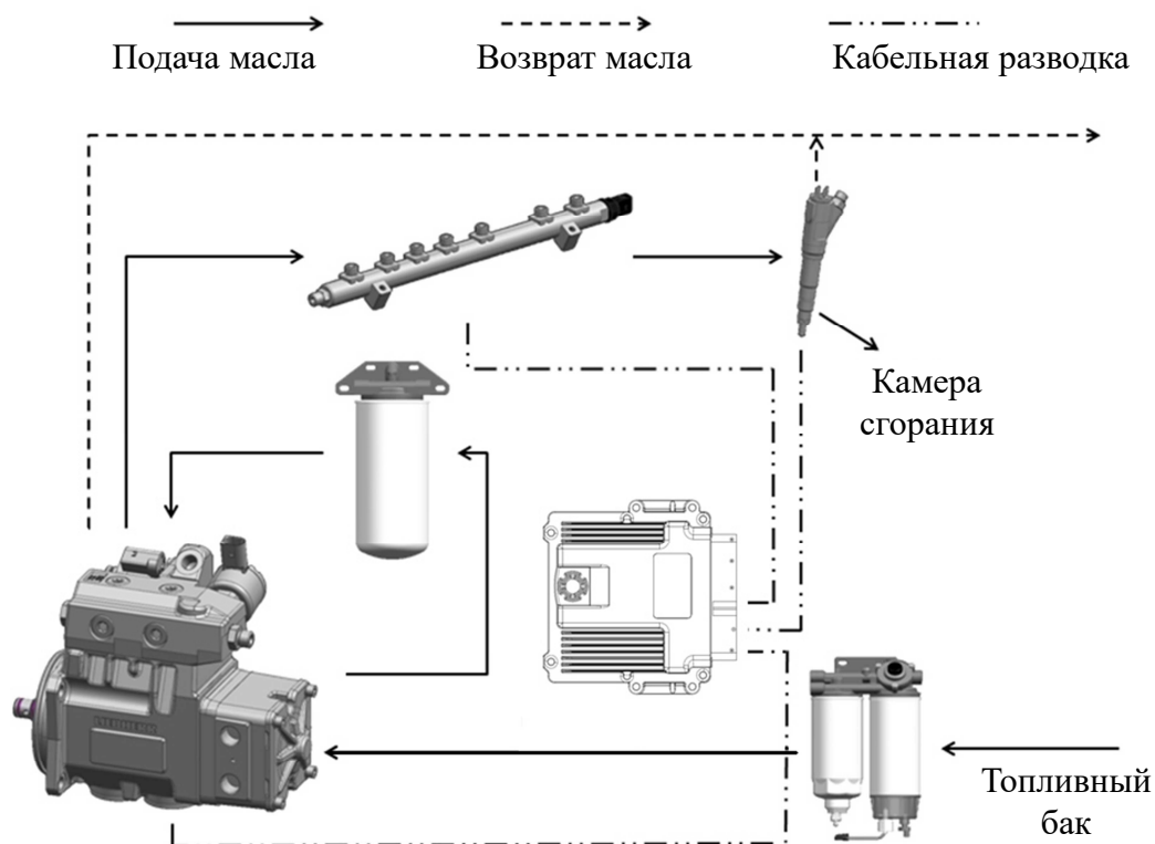
Рисунок 2-4. Схематическая диаграмма системы впрыска топлива
