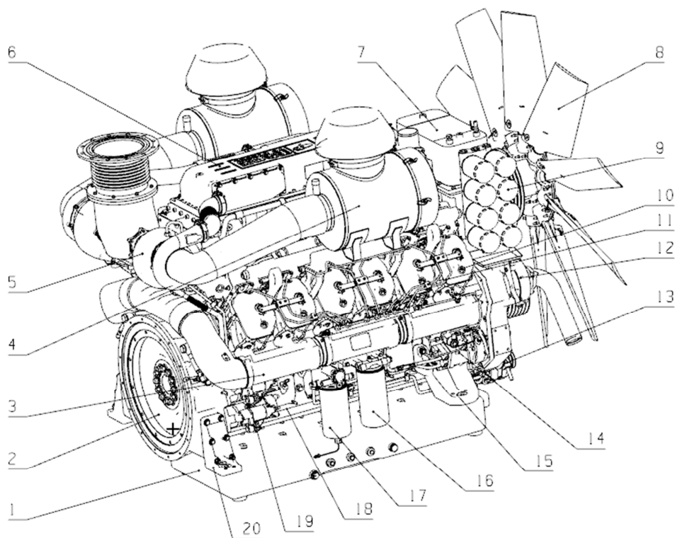
Рис. 2-2 Изометрическая проекция заднего конца двигателя
