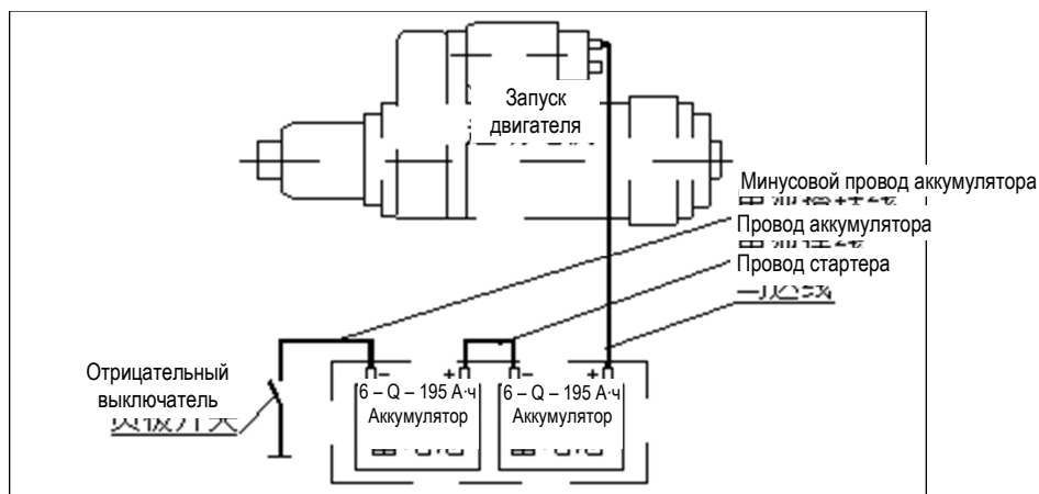
Рисунок 5-6 Схема подключения аккумулятора
