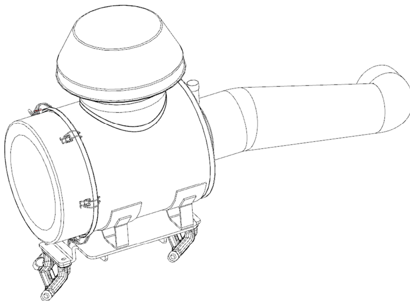
Рисунок 2-14 Воздушный фильтр
