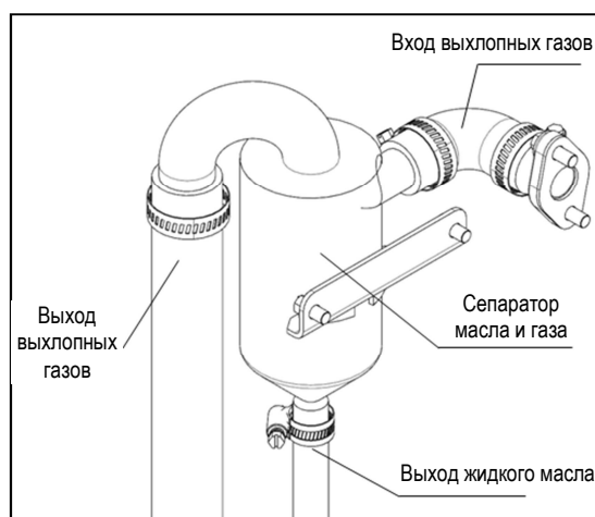
Рисунок 2-28 Структура устройства вентиляции картера
