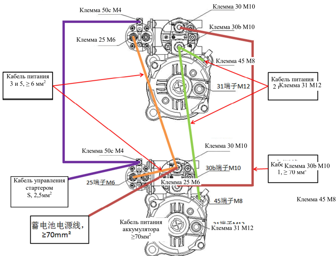
Рис. 2-13 Схема подключения стартера
