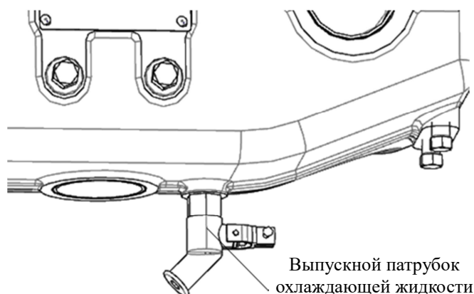
Рисунок 6-20. Отверстие для слива охлаждающей жидкости
