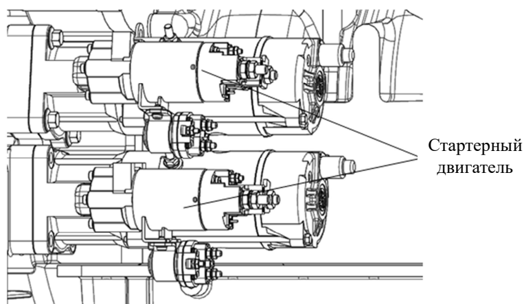
Рисунок 6-21 Проверка стартера
