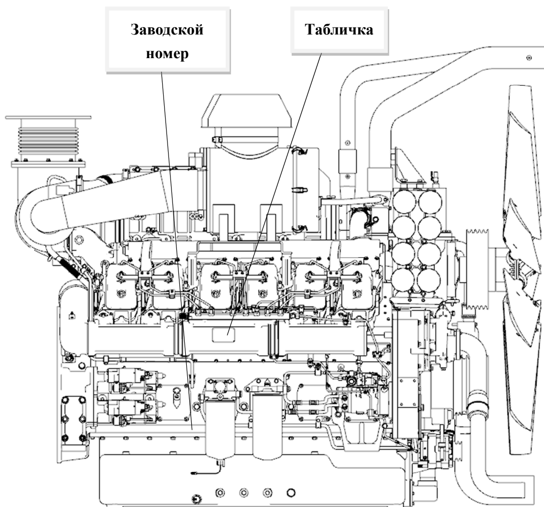
Рисунок 2-1. Маркировка двигателя и расположение заводского номера
