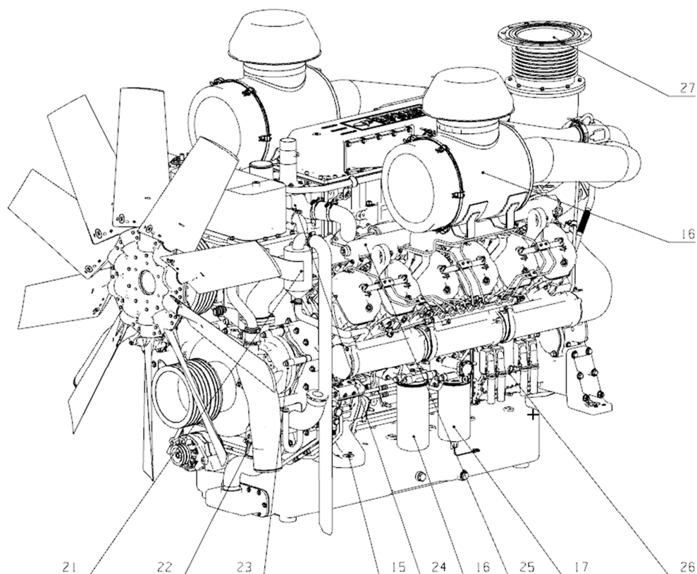
Рис. 2-3 Изометрическая проекция переднего конца двигателя
