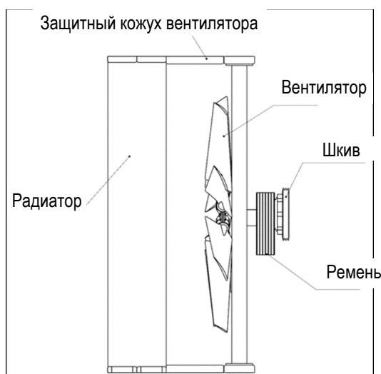
Рисунок 4-3. Требования к установке вентилятора
