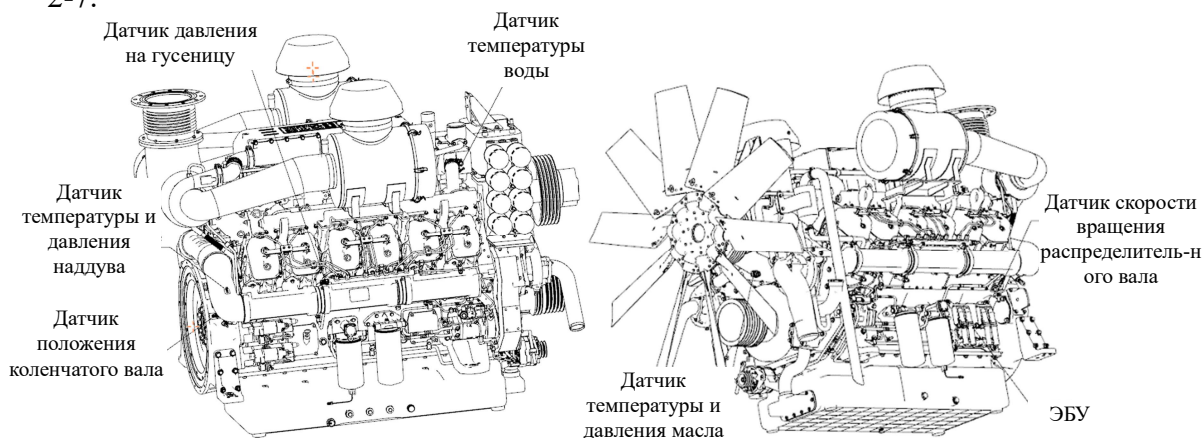
Рисунок 2-7 Расположение датчиков при установке
