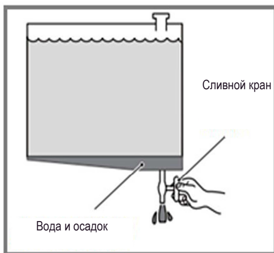
Рисунок 6-3 Дренажное отверстие топливного бака
