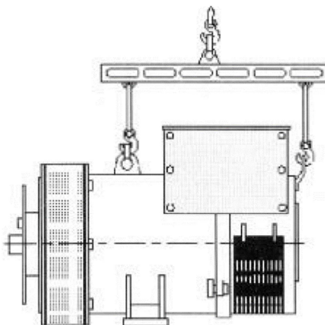
Рисунок 4-1. Подъемные проушины
