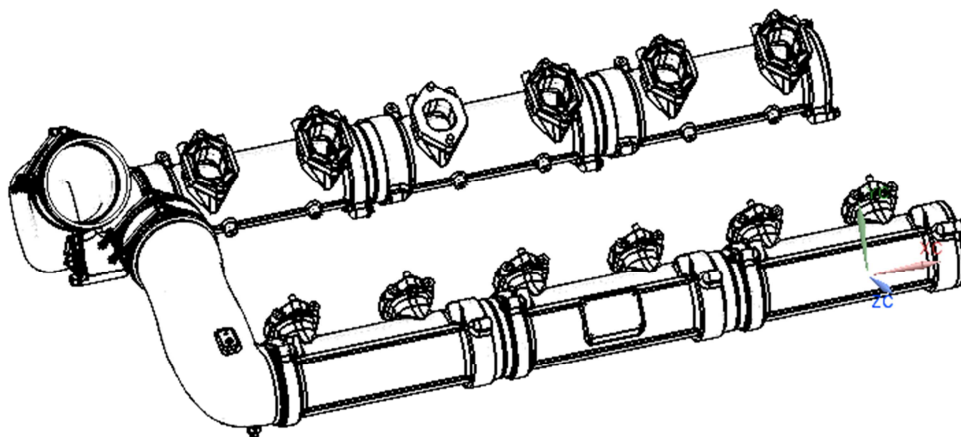
Рисунок 2-15 Узел впускного трубопровода и его установка
