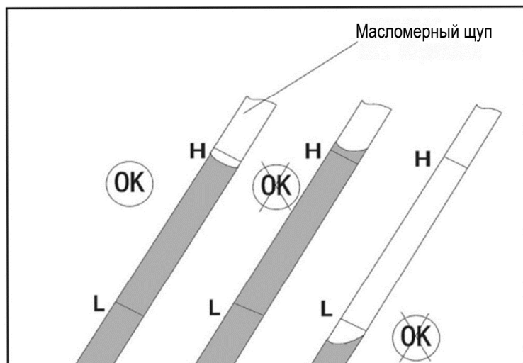
Рисунок 6-5. Различные уровни масла на масломерном щупе
