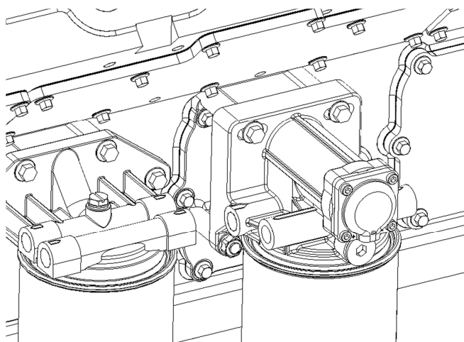
Рисунок 5-3. Удаление воздуха из топливных трубопроводов
