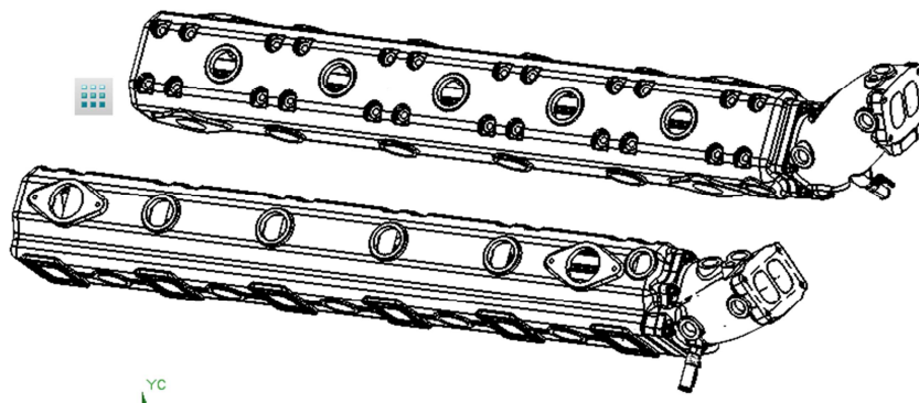
Рисунок 2-16 Выхлопная труба в сборе
