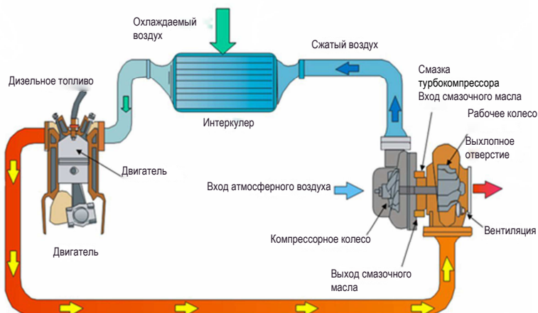
Рисунок 2-12 Принципиальная схема работы интеркулера с наддувом
