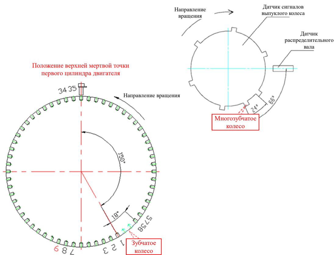
Рисунок 2-9. Взаимосвязь фаз между датчиком коленчатого вала и задающим диском демпфера
