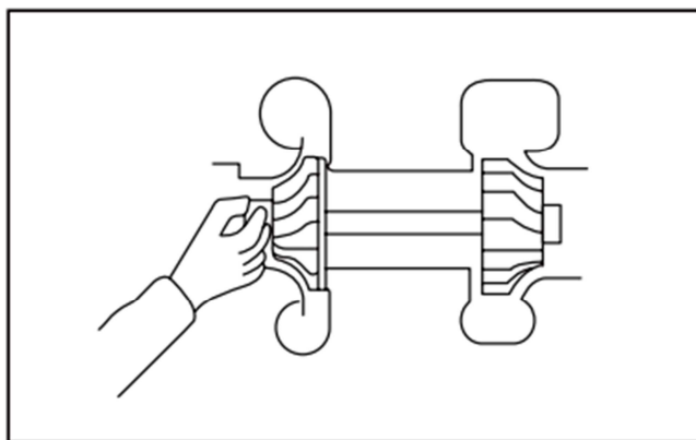
Рисунок 6-19. Проверка турбонагнетателя
