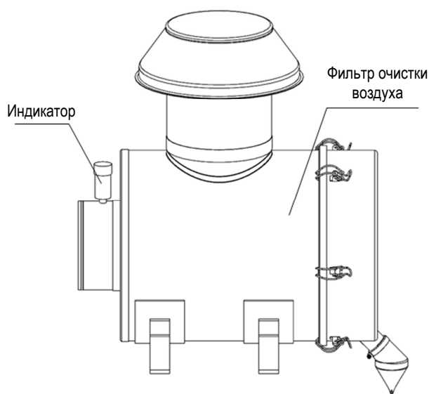
Рис. 6-6 Индикатор технического обслуживания
