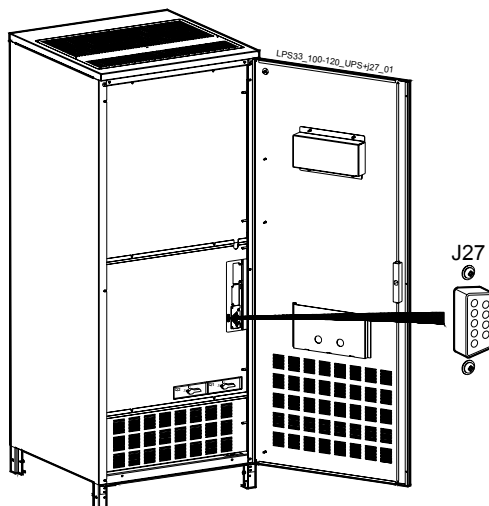
Рис. 9.1-3 Серия LP 33 / 100 - 120 кВА - Последовательный порт J27 – RS232
