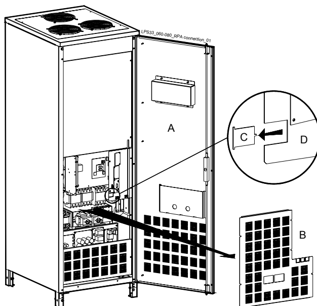
Рис. 4.8.5-2 Серия LP 33 / 60 - 80 кВА – Доступ к плате RPA
