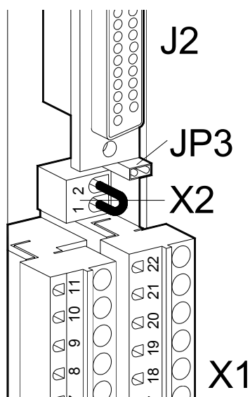
Рис. 10.2.1-2 Плата Интерфейса пользователя
