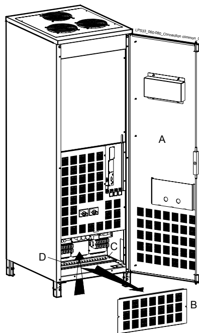
Рис. 4.8.1-3 Серия LP 33 / 60 - 80 кВА - Подключение силовых кабелей
