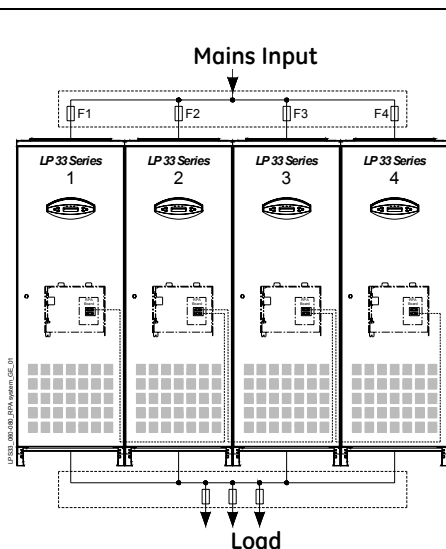
Рис. 4.7-1 Параллельная система RPA
