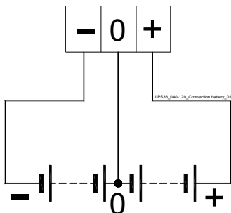
Рис. 4.8.2-4 Подключение внешней батареи
