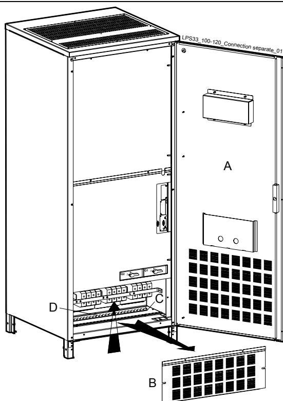
Рис. 4.8.4-2 Серия LP 33 / 100 - 120 кВА – Подключение силовых кабелей
