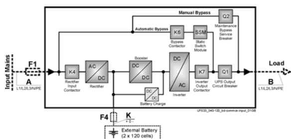
Рис. 4.8.1-1 Общее подключение электросети
