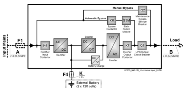
Рис. 4.7.3-1 Общие входы Выпрямителя и Байпаса
