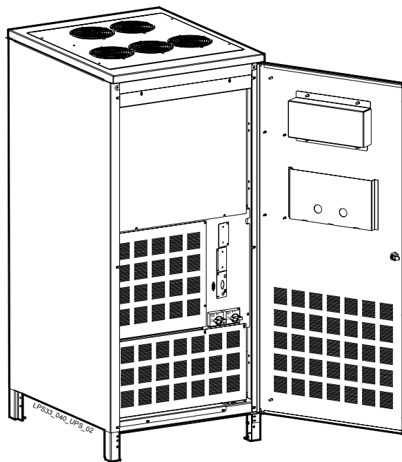
Рис. 5.1-2 Общий вид с открытой дверцей
