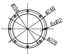
13 排气口法兰 Exhaust Flange 5:1
