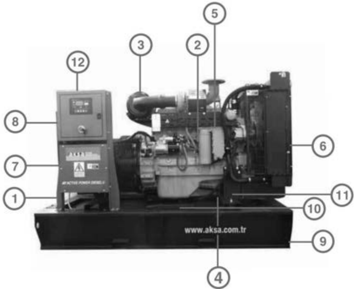
Рисунок 1 – Типовая конфигурация ДГУ
